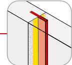
Ratkaisu liikuntasaumaan
